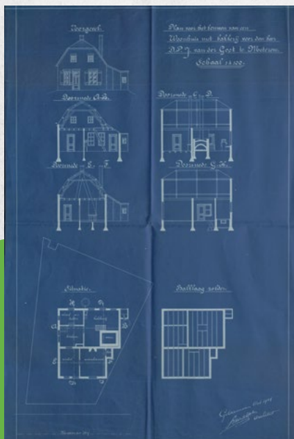
Bouwtekening bij aanvraag uit 1904 van de heer van der Goot voor het bouwen van een woonhuis met bakkerij in Meteren.
